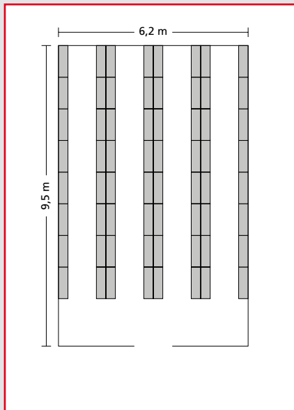
Conventioneel legbordmagazijn
