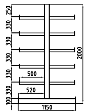
Draagarm dubbel
