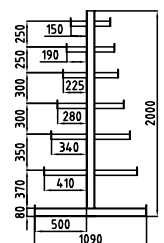
Draagarm dubbel
