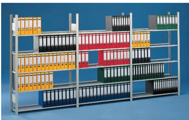
◀ Abb.: Bürosteckregal ohne Abdeckboden 3 Felder 1.250 mm Fachlänge, 1.850 mm hoch, 300 mm tief, in RAL 7035 lichtgrau
