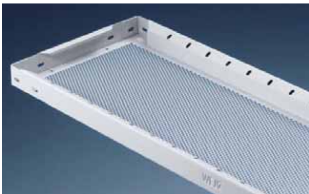
META Fachboden V 150 G mit gelochter Oberfläche
