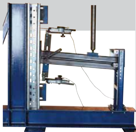
Holmanschlussversuch im META-Prüflabor: Versuchsende
