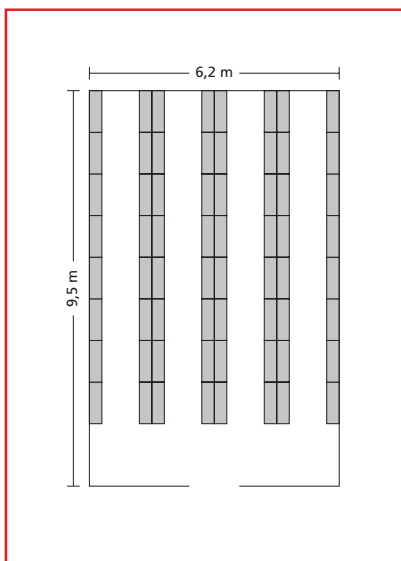
Konventionelles Fachbodenregal
