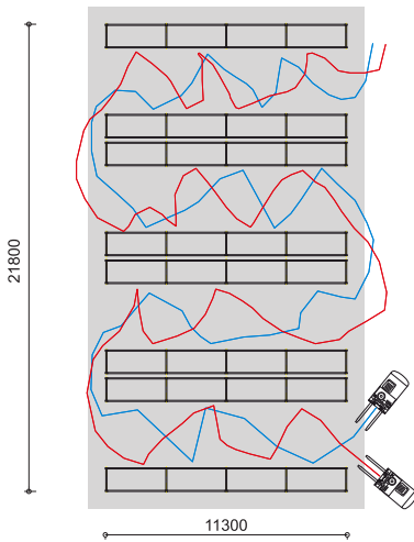
Fahrwege im konventionellen Palettenregal
