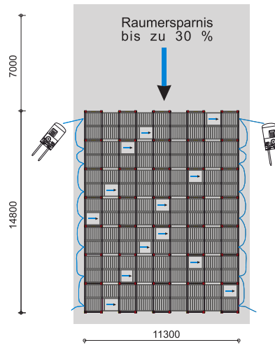
Fahrwege im META MULTILINE® S Durchlaufregal
