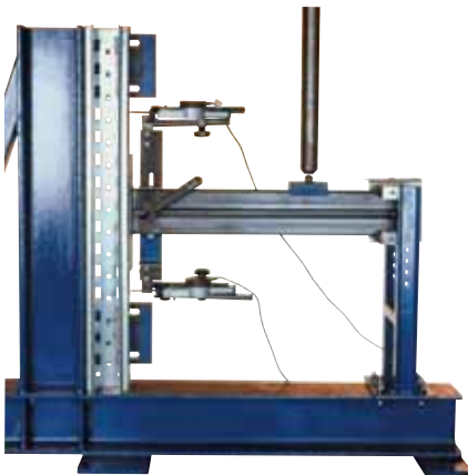
Holmanschlussversuch im META-Prüflabor: Versuchsbeginn
