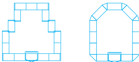
Pendeltüren-Achismaß: 800 - 1.300 mm
